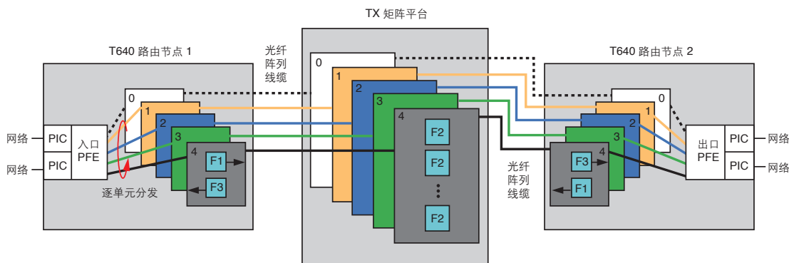
图 13：路由矩阵 Clos 交换结构的实施
